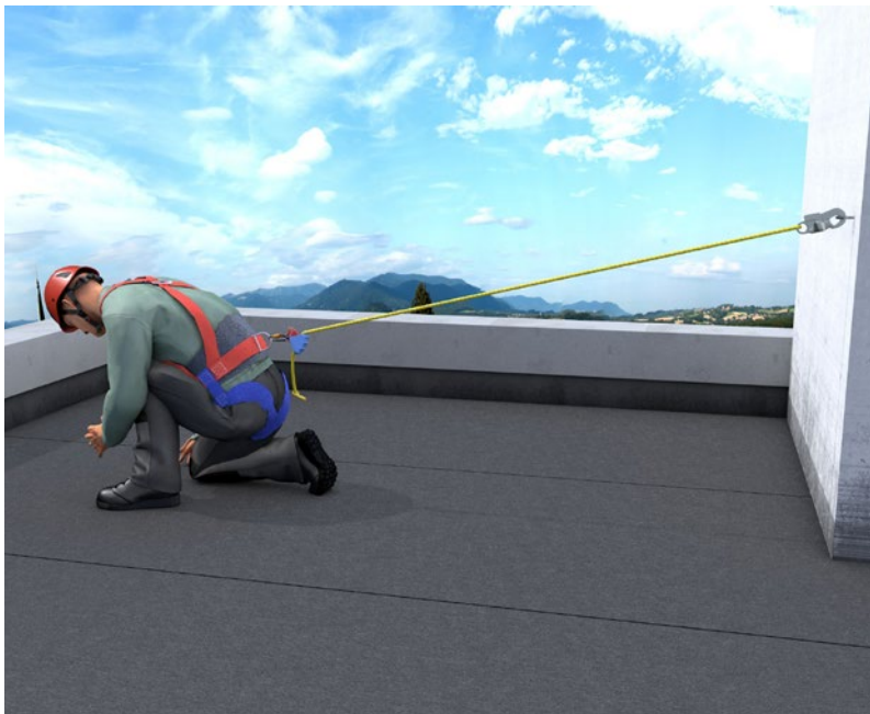
Abb. 16 Beispiel für ein Rückhaltesystem mit einstellbarer Länge, befestigt an einem Einzelanschlagpunkt
